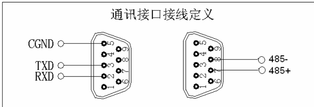
图6.4 通讯接线图
