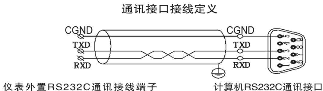
图 7.1 RS-232C 通讯接线方法
