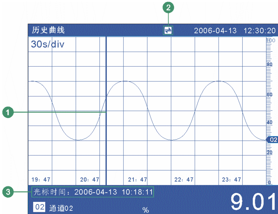
图 5.6 历史曲线追忆画面
