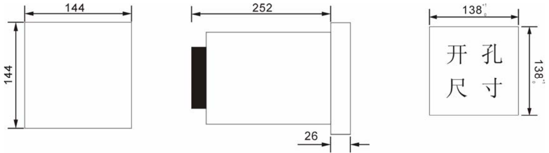
图6.1 仪表外形尺寸，安装方法及开孔尺寸
