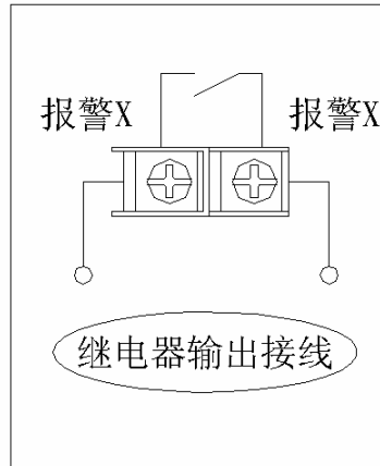
图6.3 继电器触点输出接线图
