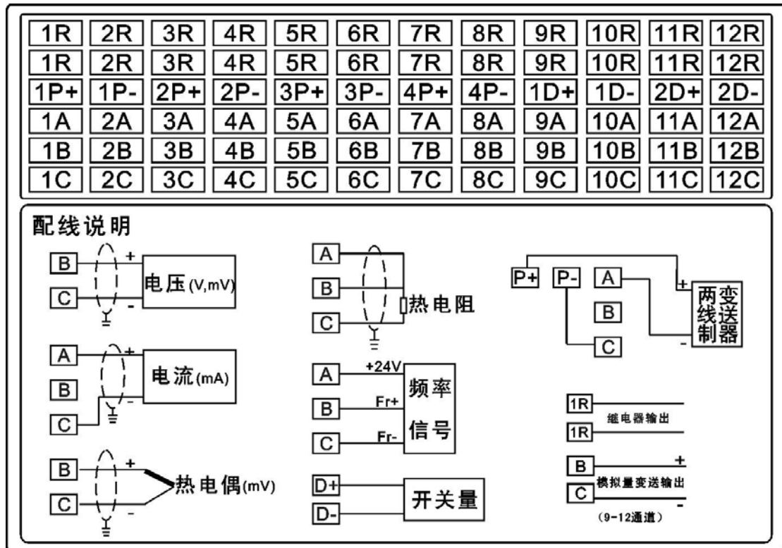
图6.2 端子及接线图
