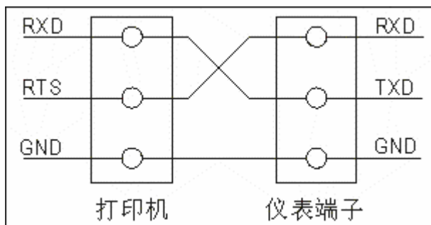
图 5.9 打印机接线图
